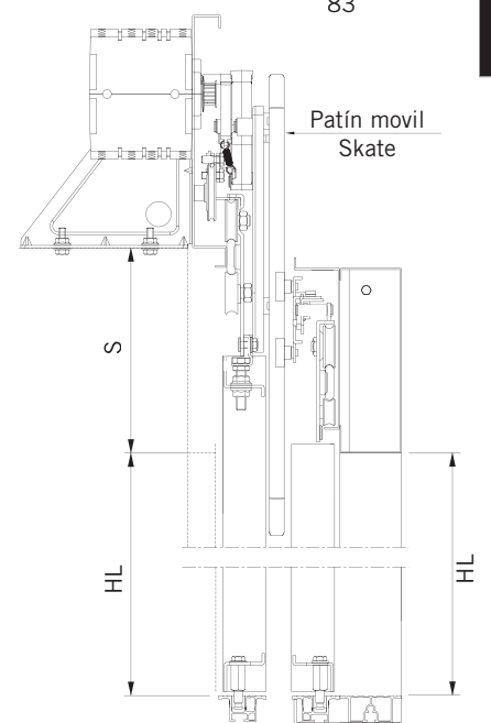
D: Patín modelo Q para desplazamientos superiores a 150 mm. D: Q model skate for upper displacements than 150 mm.
