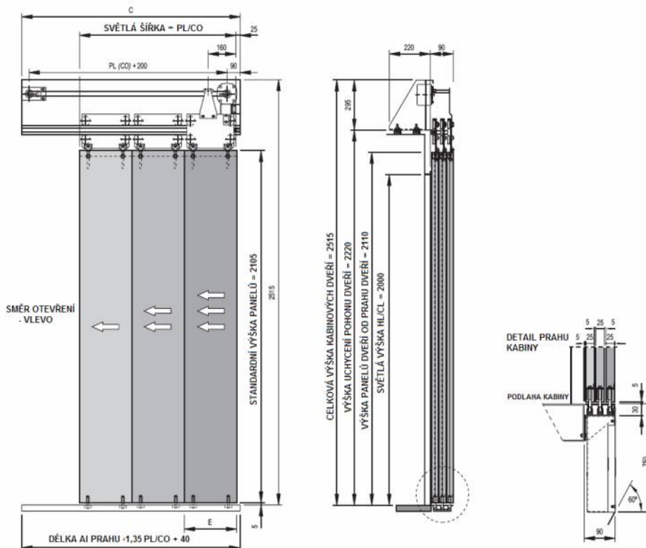
SPŘAŽENÍ S LEVÝMI RUČNÍMI ŠACHETNÍMI DVEŘMI
